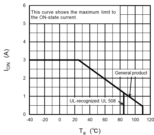
Fig. 16.1.2 I_{ON} - T_a
