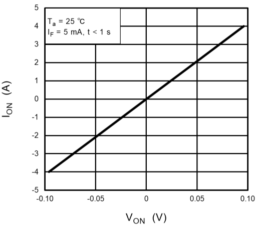
Fig. 16.1.4 I_{ON} - V_{ON}
