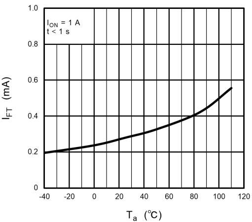
Fig. 16.1.6 I_{FT} - T_a
