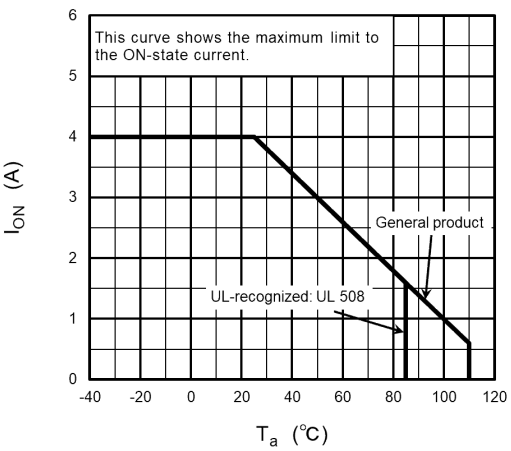
Fig. 16.1.2 I_{ON} - T_a
