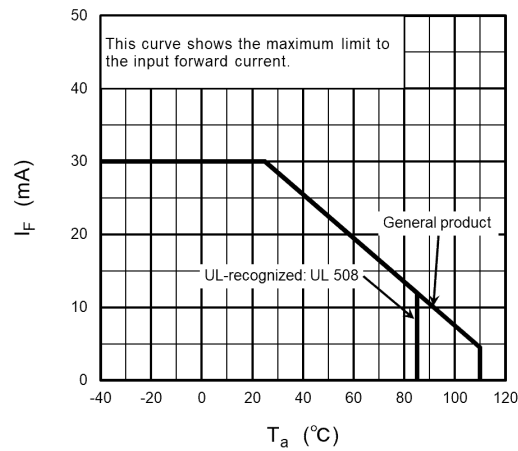
Fig. 16.1.1 I_F - T_a
