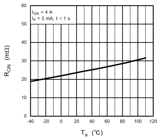
Fig. 16.1.5 R_{ON} - T_a
