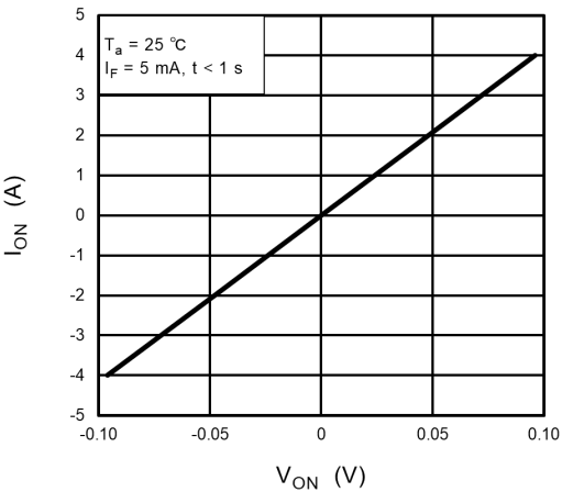
Fig. 16.1.4 I_{ON} - V_{ON}
