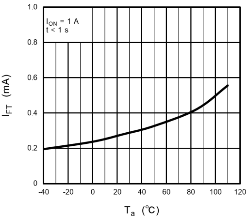
Fig. 16.1.6 I_{FT} - T_a
