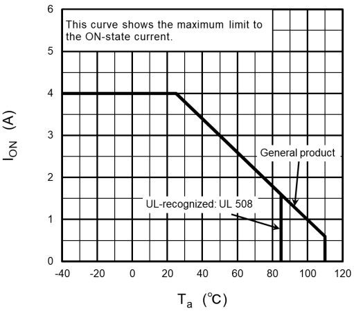
Fig. 16.1.2 I_{ON} - T_a
