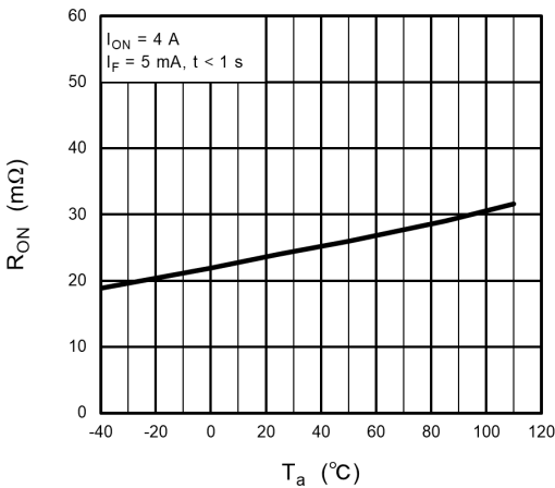
Fig. 16.1.5 R_{ON} - T_a
