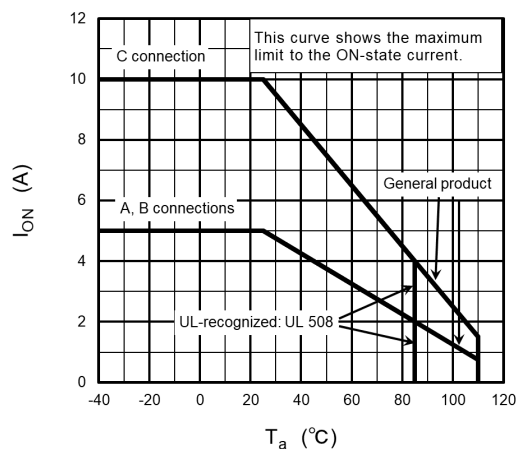
Fig. 16.1.2 I_{ON} - T_a
