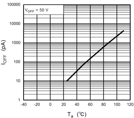
Fig. 12.10 I_{OFF} - T_a
