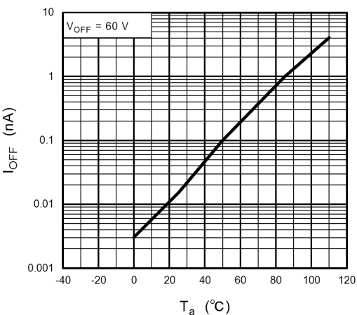
Fig. 12.10 I_{OFF} - T_a
