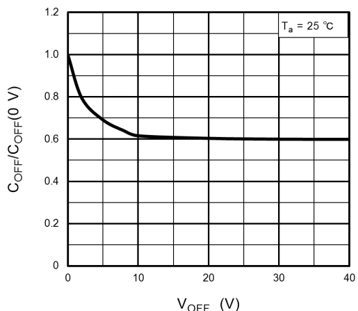
Fig. 12.11 C_{OFF} - V_{OFF}
