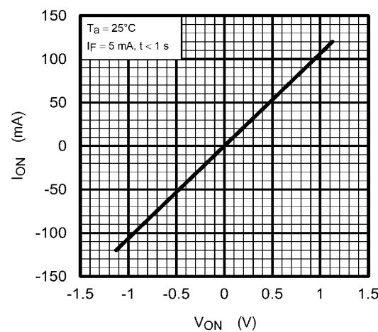
Fig. 12.4 I_{ON} - V_{ON}
