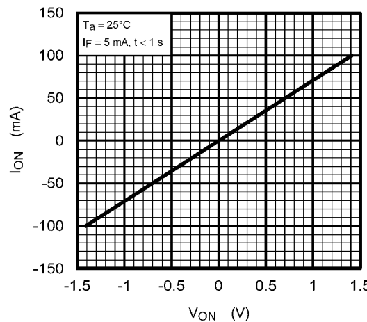
Fig. 12.4 I_{ON} - V_{ON}
