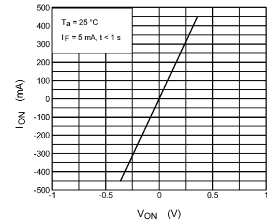
Fig. 12.4 I_{ON} - V_{ON}
