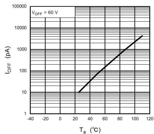
Fig. 12.8 I_{OFF} - T_a
