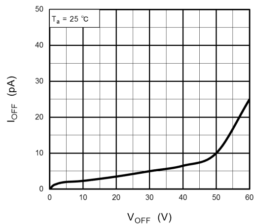
Fig. 12.7 I_{OFF} - V_{OFF}
