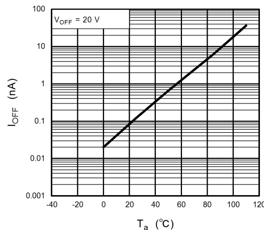
Fig. 12.10 I_{OFF} - T_a
