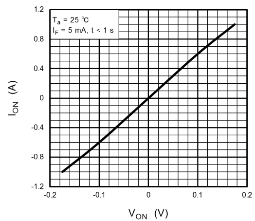
Fig. 12.4 I_{ON} - V_{ON}
