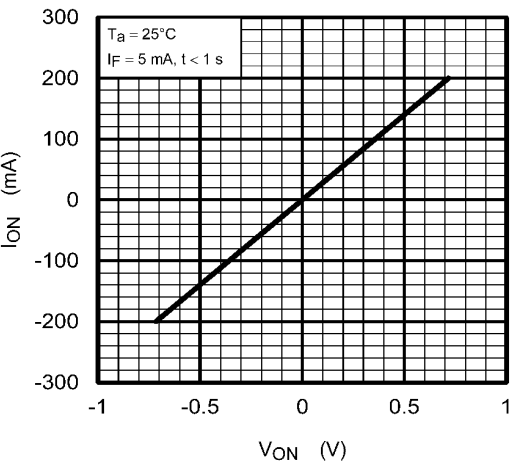
Fig. 12.1.4 I_{ON} - V_{ON}
