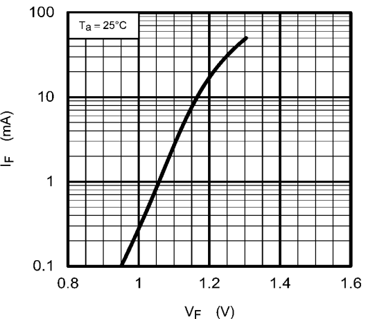
Fig. 12.1.3 I_F - V_F
