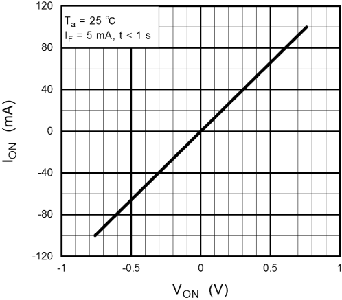
Fig. 12.1.4 I_{ON} - V_{ON}
