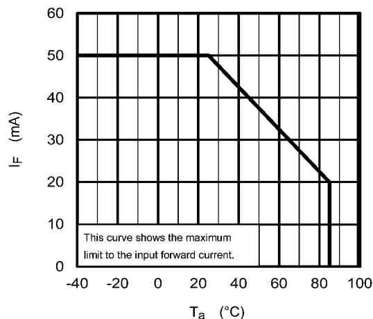
Fig. 12.1.1 I_F - T_a
