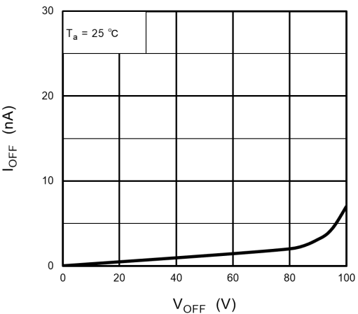
Fig. 12.10 I_{OFF} - V_{OFF}
