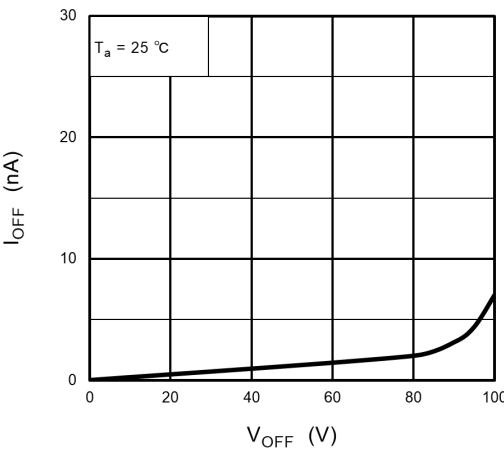
Fig. 12.10 I_{OFF} - V_{OFF}
