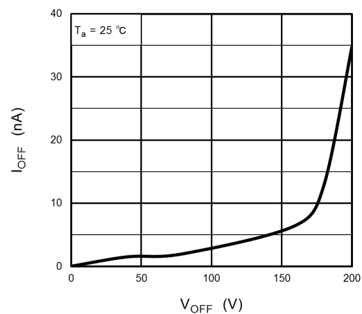
Fig. 12.10 I_{OFF} - V_{OFF}
