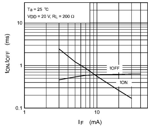
Fig. 12.8 tON,tOFF - IF
