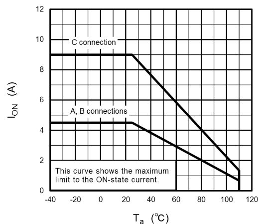
Fig. 12.1.2 I_{ON} - T_a
