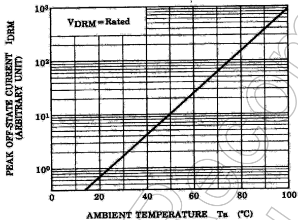
NORMALIZED I_{DRM} - T_a
