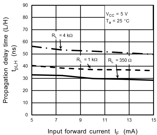
Fig. 13.2.20 t_{pLH} - I_F
