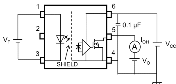
Fig. 13.1.1 I_{OH} Test Circuit
