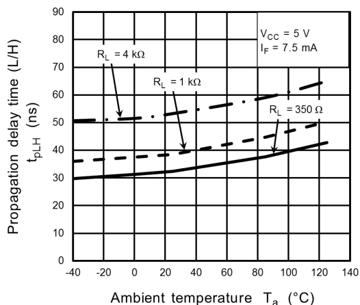
Fig. 13.2.14 t_{pLH} - T_a
