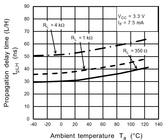
Fig. 13.2.17 t_{pLH} - T_a
