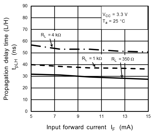
Fig. 13.2.23 t_{pLH} - I_F
