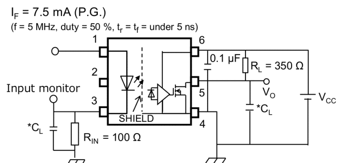
Fig. 13.1.5 I_{FHL} , I_{FLH} , I_{HYS} Test Circuit
