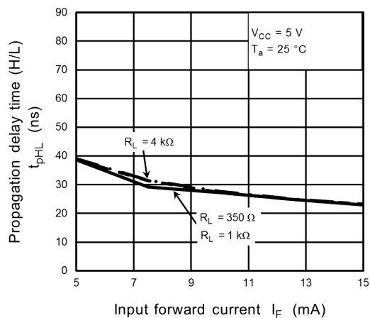
Fig. 13.2.19 t_{pHL} - I_F
