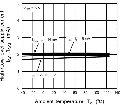
Fig. 14.2.6 I_{CCH} / I_{CCL} - T_a
