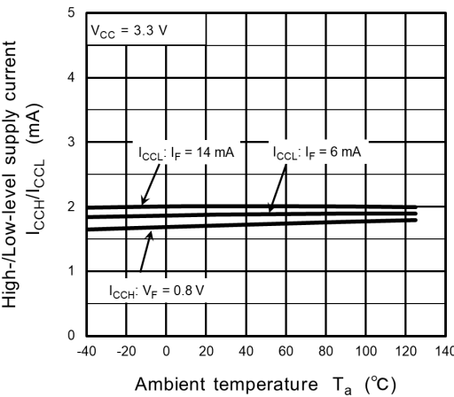
Fig. 14.2.5 I_{CCH} / I_{CCL} - T_a
