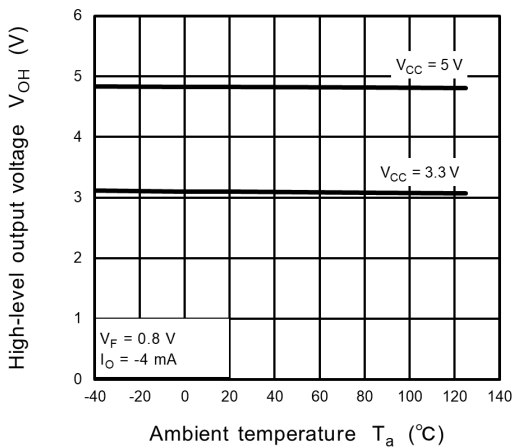
Fig. 14.2.4 V_{OH} - T_a
