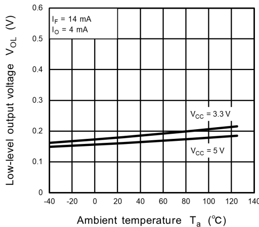
Fig. 14.2.3 V_{OL} - T_a
