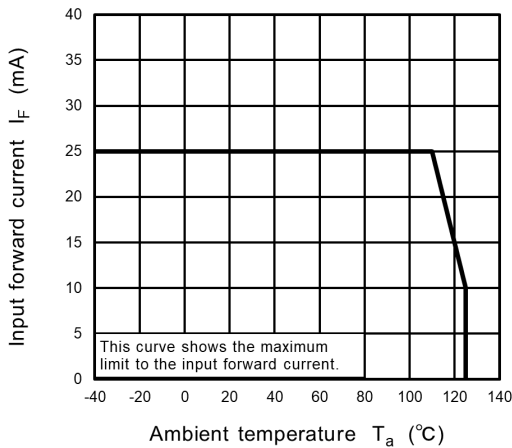
Fig. 14.2.2 I_F - T_a
