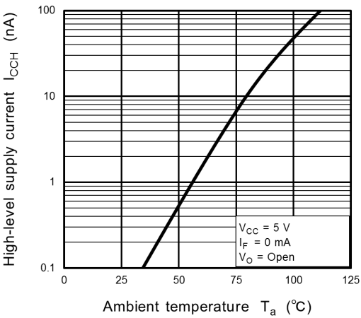
Fig. 12.2.4 I_{CCH} - T_a
