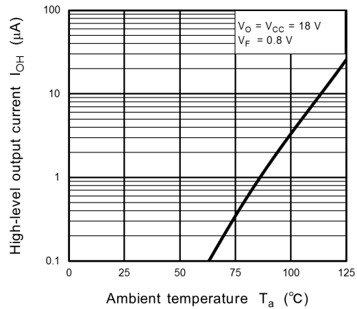
Fig. 12.2.3 I_{OH} - T_a
