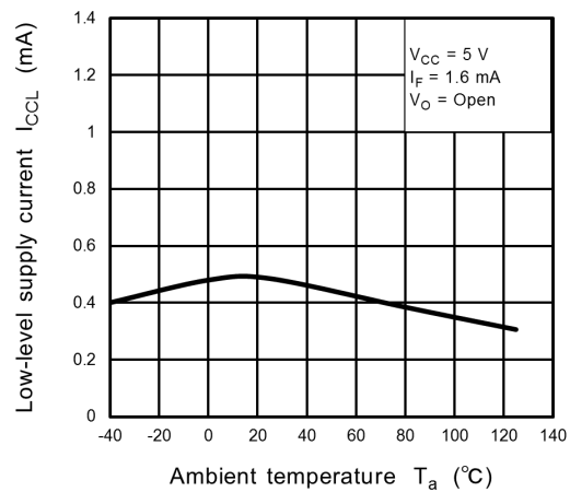
Fig. 12.2.5 I_{CCL} - T_a
