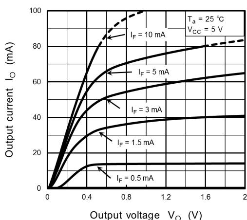
Fig. 12.2.11 I_O - V_O
