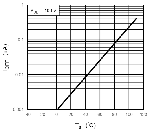
Fig. 14.9 I_{OFF} - T_a
