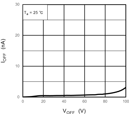
Fig. 14.10 I_{OFF} - V_{OFF}
