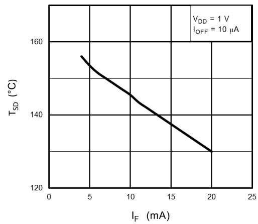
Fig. 14.14 T_{SD} - I_F
