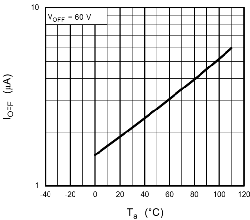
Fig. 14.11 I_{OFF} - T_a
