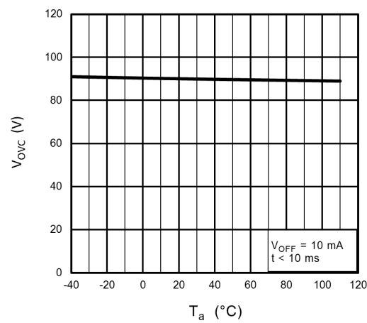
Fig. 14.15 V_{OVC} - T_a
