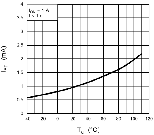
Fig. 14.8 I_{FT} - T_a
