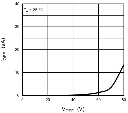
Fig. 14.12 I_{OFF} - V_{OFF}
