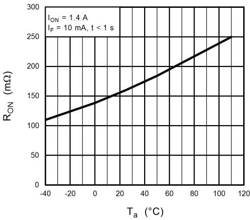
Fig. 14.7 R_{ON} - T_a
