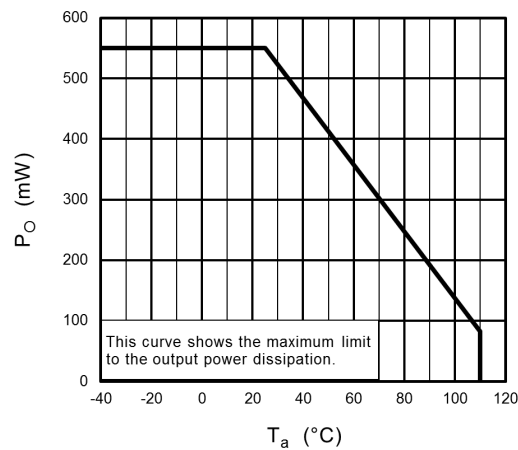
Fig. 14.4 P_O - T_a
