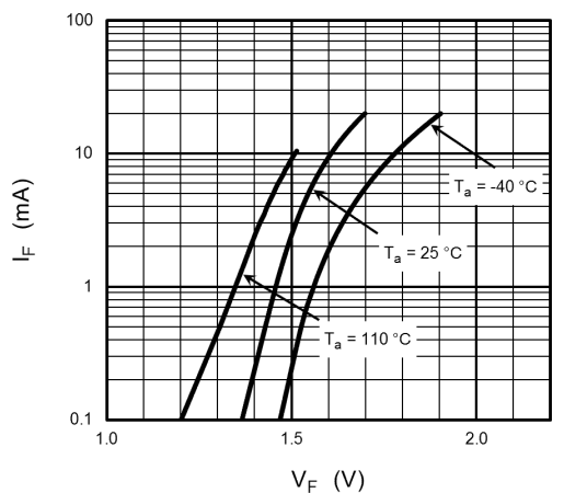
Fig. 14.5 I_F - V_F
