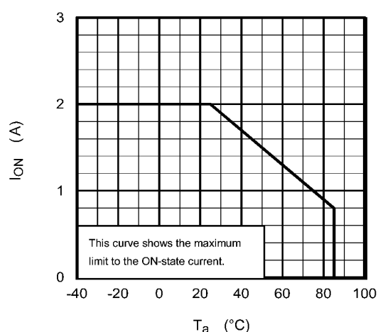
Fig. 16.2 I_{ON} - T_a
