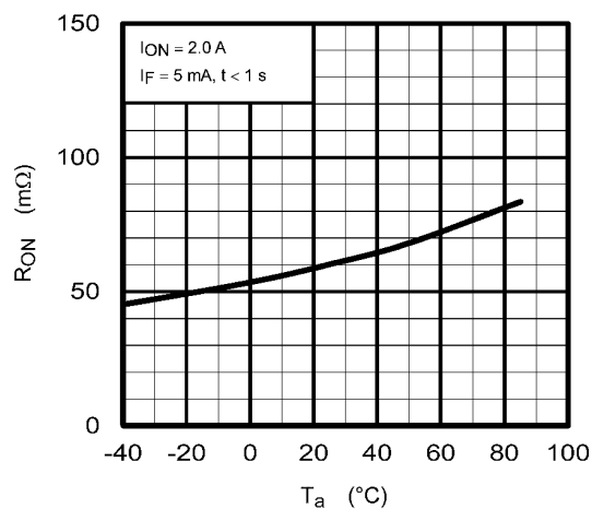
Fig. 16.5 R_{ON} - T_a
