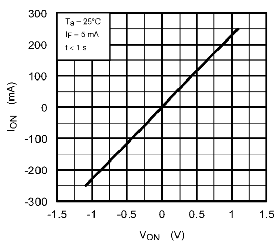
Fig. 16.4 I_{ON} - V_{ON}
