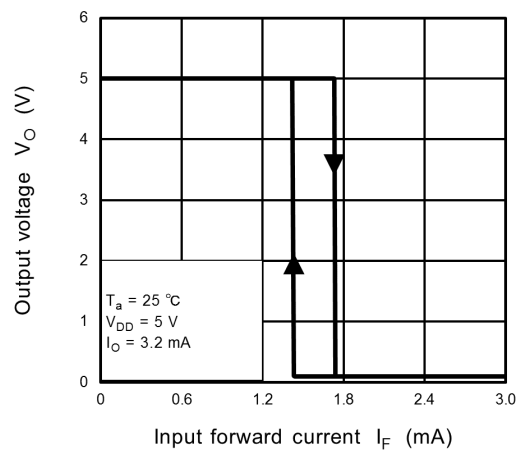
Fig. 12.2.11 V_O - I_F
