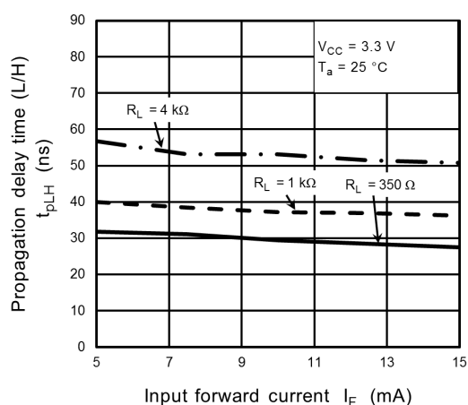
Fig. 12.2.23 t_{pLH} - I_F
