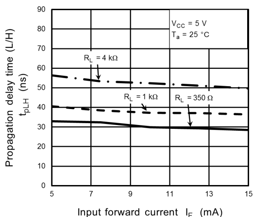
Fig. 12.2.20 t_{pLH} - I_F
