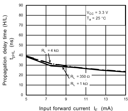
Fig. 12.2.22 t_{pHL} - I_F
