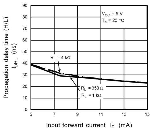
Fig. 12.2.19 t_{pHL} - I_F
