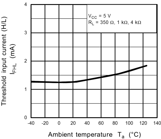
Fig. 12.2.7 I_{FHL} - T_a
