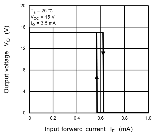
Fig. 12.2.13 V_O - I_F
