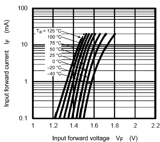
Fig. 12.2.1 I_F - V_F
