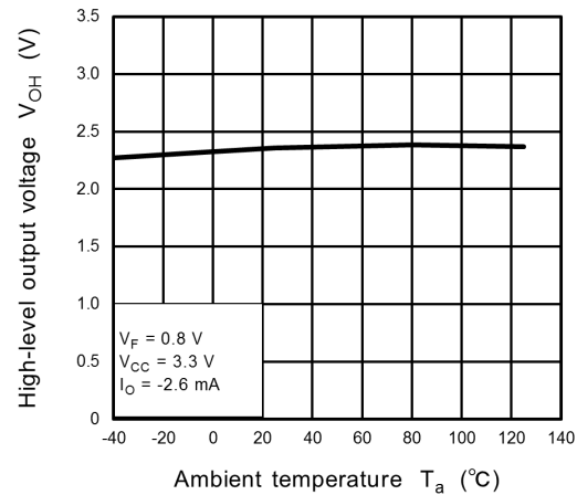
Fig. 12.2.4 V_{OH} - T_a
