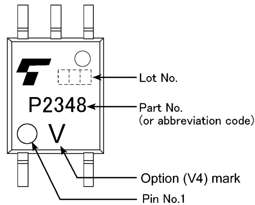
Fig. 16.4 Marking Example(Note)
