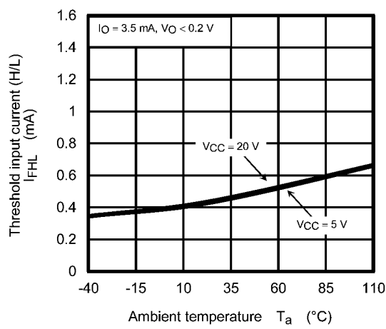
Fig. 12.2.2 I_{FHL} - T_a
