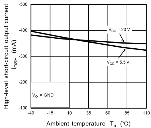
Fig. 12.2.10 I_{OH} - T_a
