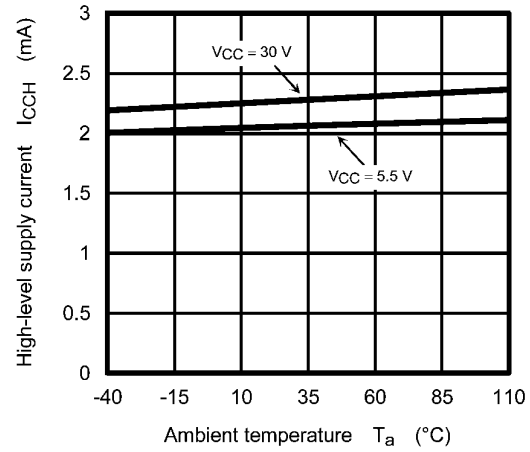
Fig. 12.2.8 I_{CCH} - T_a
