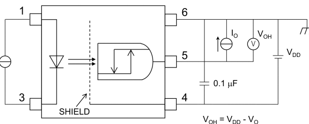
Fig. 12.1.2 V_{OH} Test Circuit
