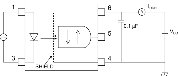
Fig. 12.1.4 I_{DDH} Test Circuit
