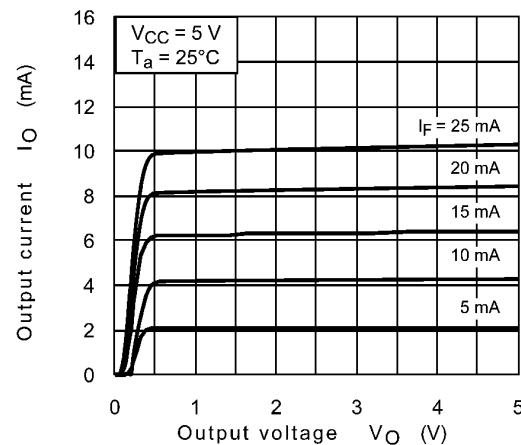
Fig. 12.2.11 I_O - V_O
