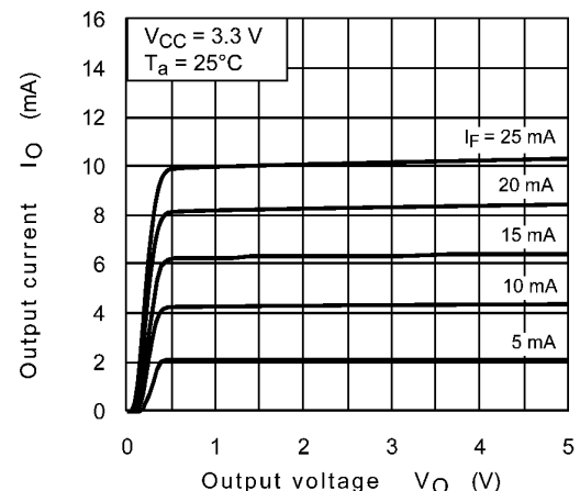
Fig. 12.2.12 I_O - V_O
