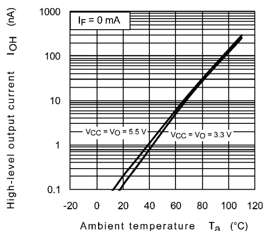
Fig. 12.2.2 I_{OH} - T_a
