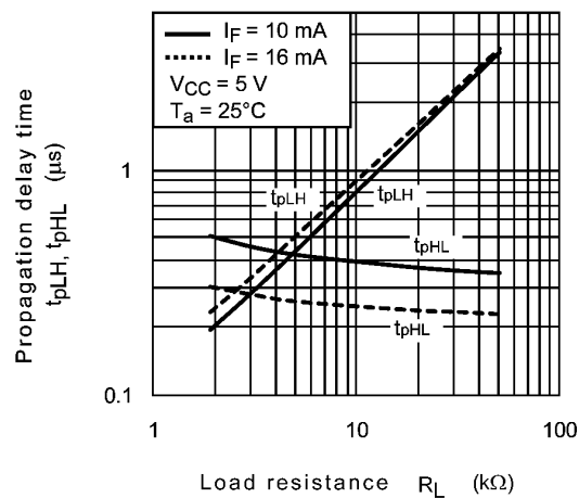
Fig. 12.2.19 t_{pLH} , t_{pHL} - R_L
