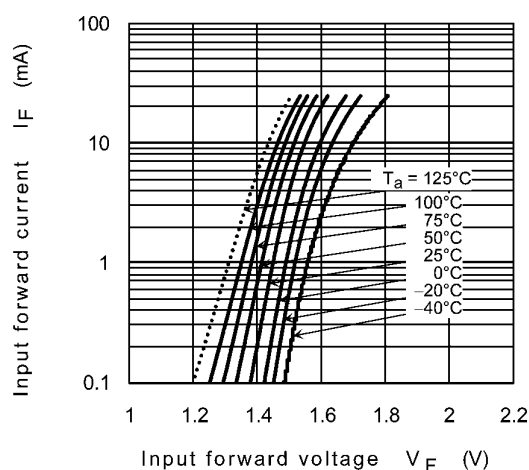
Fig. 12.2.1 I_F - V_F
