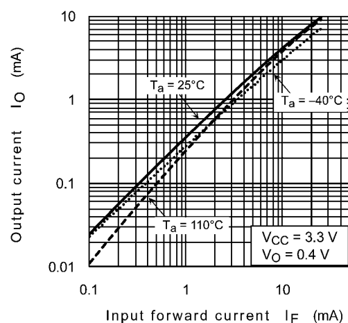
Fig. 12.2.5 I_O - I_F
