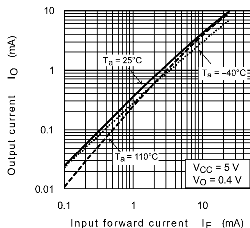
Fig. 12.2.3 I_O - I_F
