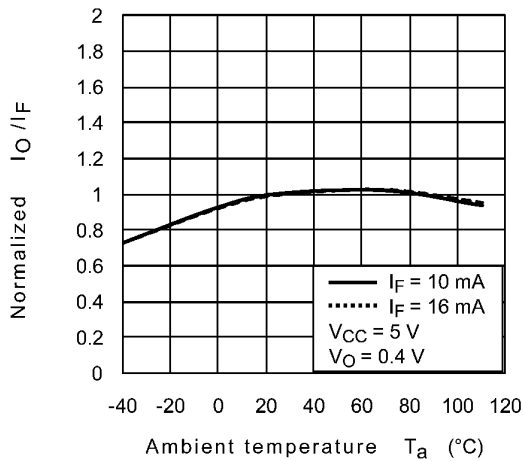
Fig. 12.2.8 I_O/I_F - T_a
