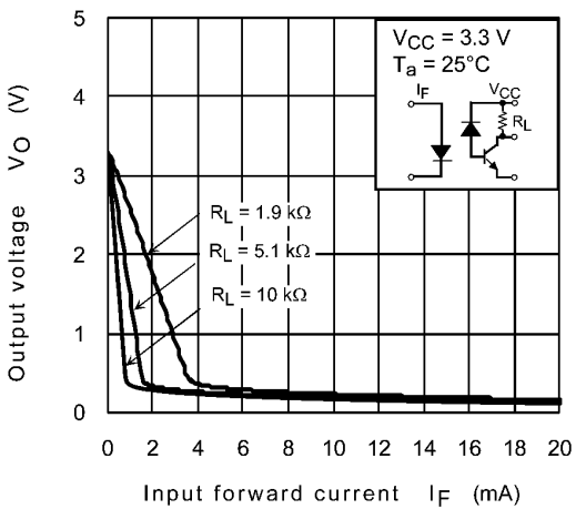
Fig. 12.2.14 V_O - I_F
