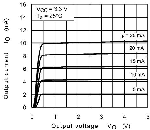
Fig. 12.2.12 I_O - V_O
