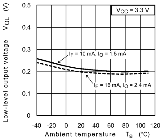
Fig. 12.2.16 V_{OL} - T_a
