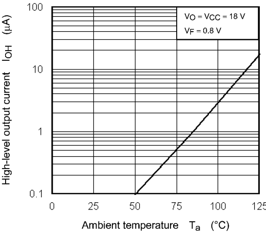
Fig. 12.2.3 I_{OH} - T_a
