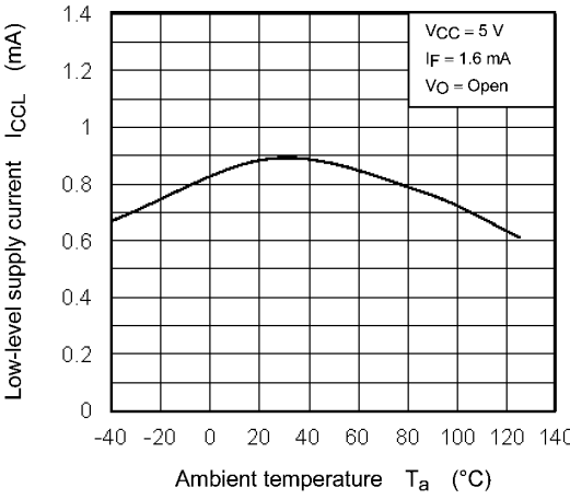
Fig. 12.2.5 I_{CCL} - T_a
