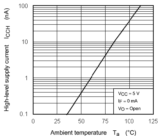
Fig. 12.2.4 I_{CCH} - T_a
