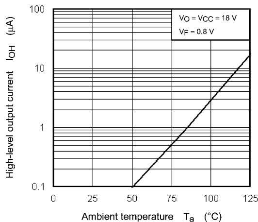
Fig. 12.2.3 I_{OH} - T_a
