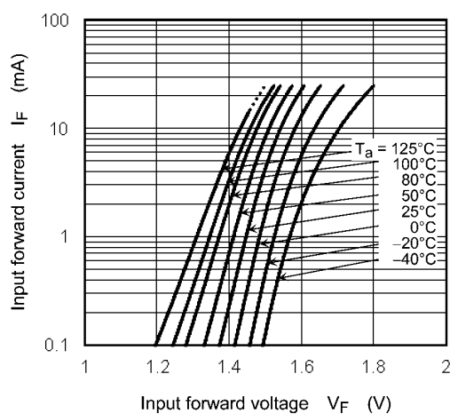
Fig. 12.2.1 I_F - V_F
