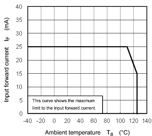
Fig. 12.2.2 I_F - T_a
