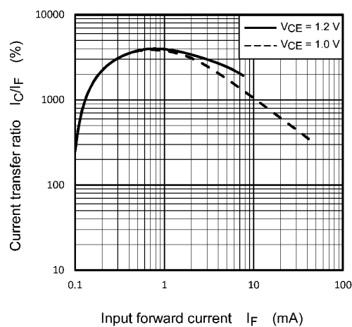
Fig. 11.10 I_C/I_F - I_F
