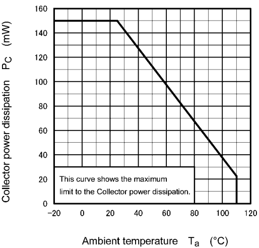
Fig. 11.2 P_C - T_a
