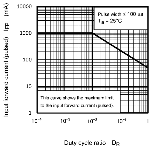
Fig. 11.3 I_{FP} - D_R
