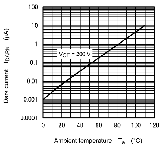
Fig. 11.9 I_{DARK} - T_a
