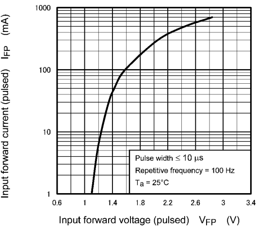
Fig. 11.6 I_{FP} - V_{FP}
