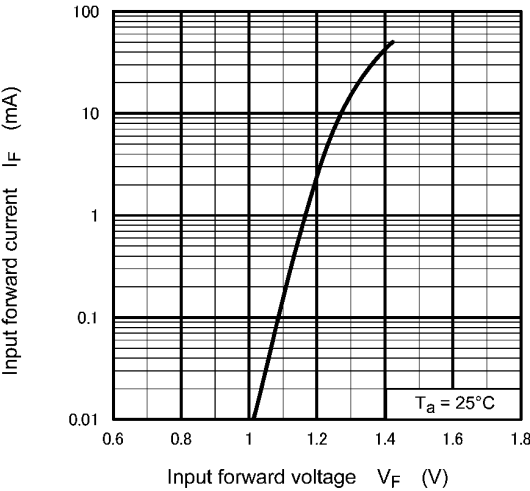
Fig. 11.4 I_F - V_F
