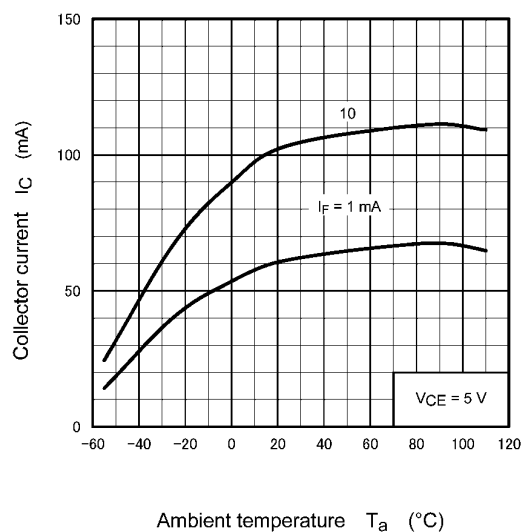
Fig. 11.12 I_C - T_a
