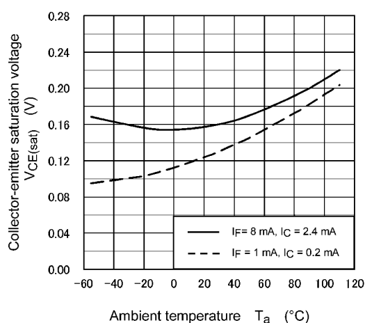
Fig. 11.12 V_{CE(\text{sat})} - T_a
