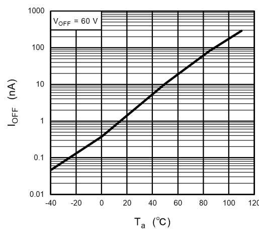
Fig. 14.1.9 I_{OFF} - T_a
