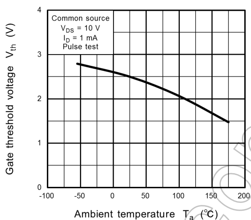
Fig. 9.9 V_{th} - T_a
