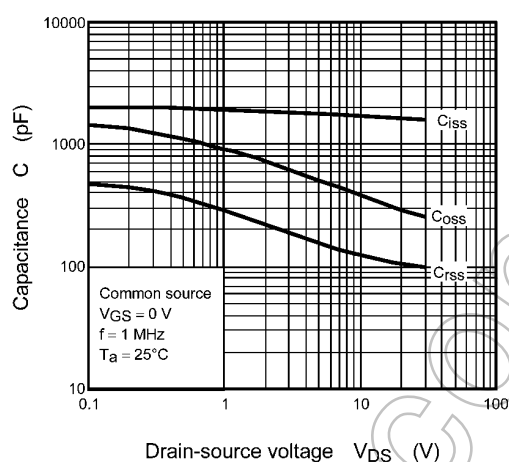
Fig. 8.9 Capacitance - V_{DS}
