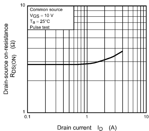
Fig. 8.6 R_{DS(ON)} - I_D
