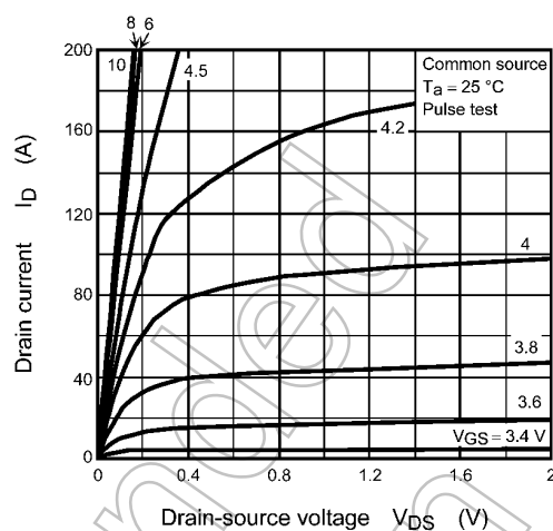
Fig. 9.2 I_D - V_{DS}
