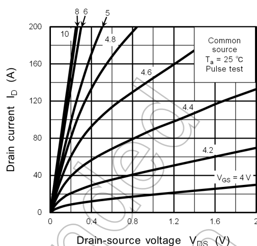
Fig. 9.2 I_D - V_{DS}
