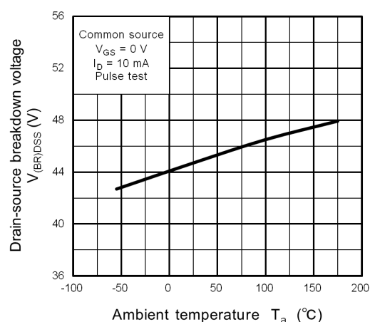
Fig. 8.12 V_{(BR)DSS} - T_a
