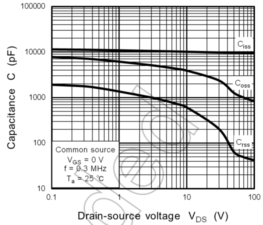
Fig. 9.8 Capacitance - V_{DS}
